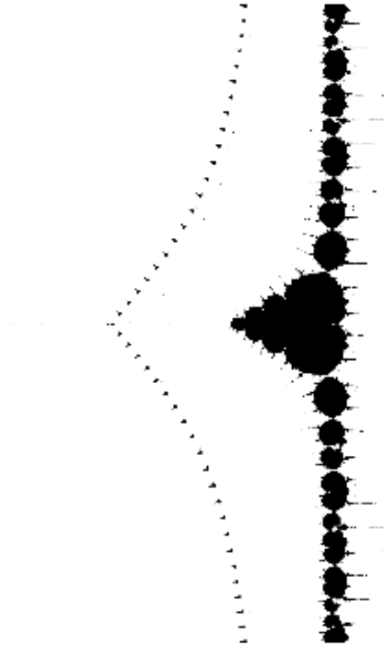
FIG. 1.1: A_\phi
